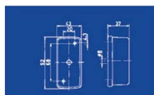
PILOTO LATERAL BLANCO-ROJO SIN TORNILLOS ref. 172231
