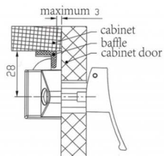
CIERRE TIRADOR CROMO ref. 152051C
