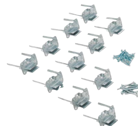
KIT INSTALACION DOMETIC MIDI HEKI WS53-60 MM ref. 144531.01 Kit de montaje que incluye soportes y tornillos para un montaje fácil y sin problemas de las claraboyas Midi Heki o Midi Heki Style.
