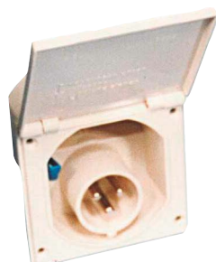
TOMA CORRIENTE 220V CUADRADA CEE ref. 170115
