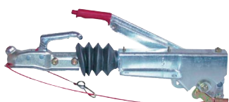
CONJUNTO ENGANCHE AK161 - 1000 KG ref. 130110
