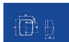
PILOTO JOKON LATERAL BLANCO-ROJO ref. 172232
