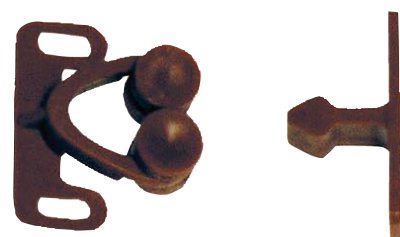
Se sirve en Bolsas de 10 unidades CIERRE PRESIÓN DOBLE RODILLO INTERIOR ref. 152060
