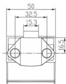
CIERRE TIRADOR NEGRO ref. 152051N
